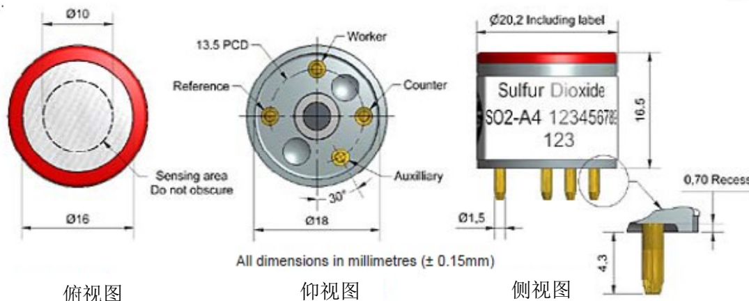
图1 SO2-A4示意图
